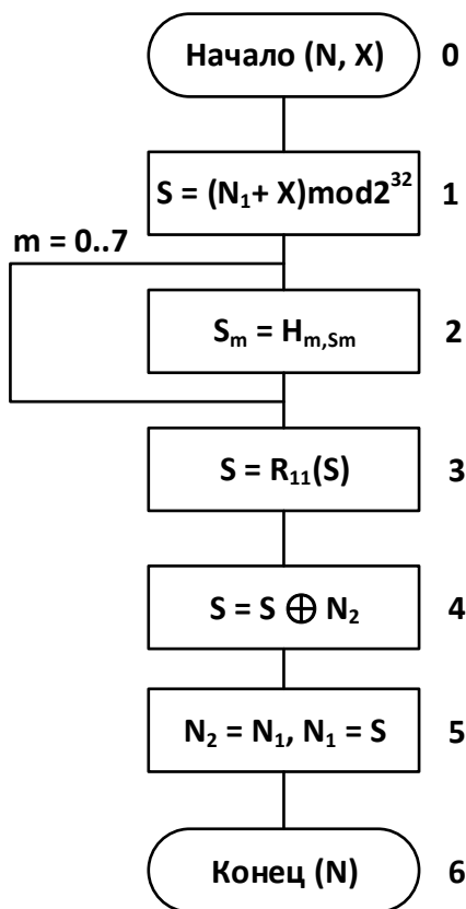
Рис. 1. Схема основного шага криптопреобразования алгоритма ГОСТ 28147-89
