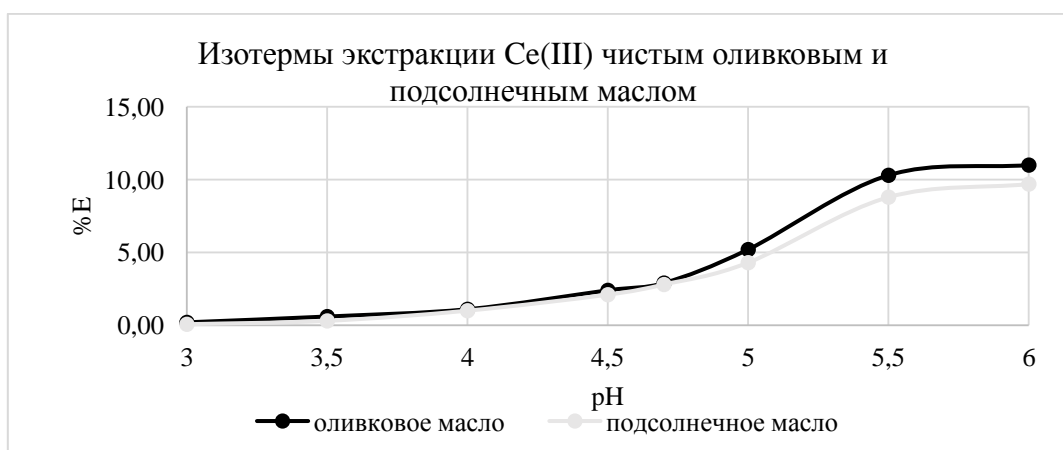
Рис. 2. Зависимость степени извлечения Се (III) от равновесного pH водной фазы при экстракции оливковым и подсолнечным маслом без добавления олеиновой кислоты
