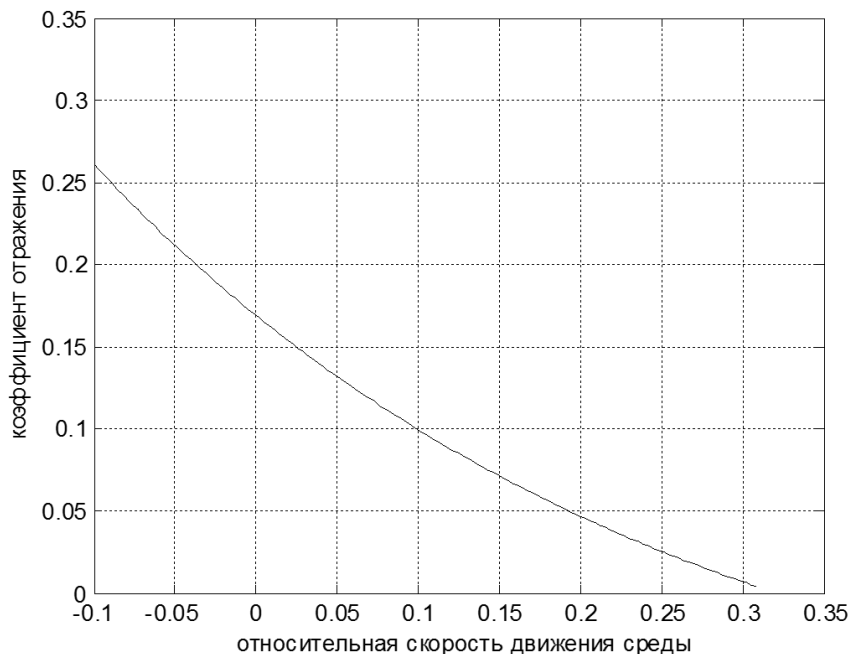
Рис. 3. Коэффициент отражения ( \rho_2/\rho_1 = 1,1; u/c_1 = 0,1, c_2/c_1 = 1,2 )
